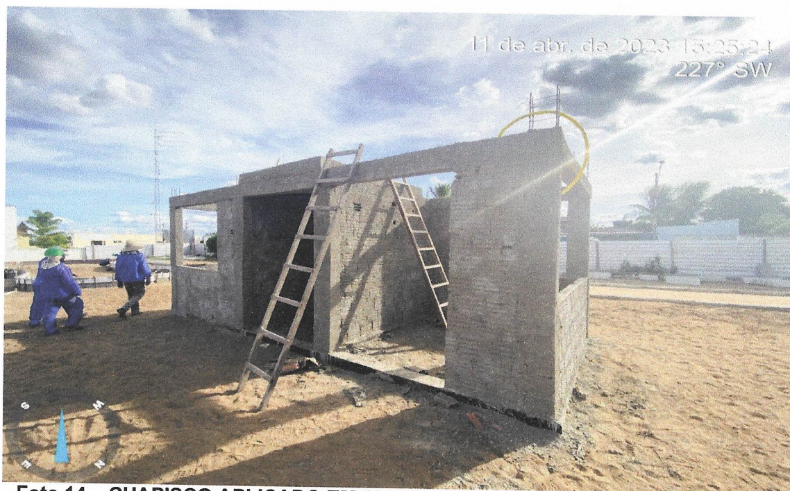
Foto 14 – CHAPISCO APLICADO EM ALVENARIA (COM PRESENÇA DE VÃOS)
